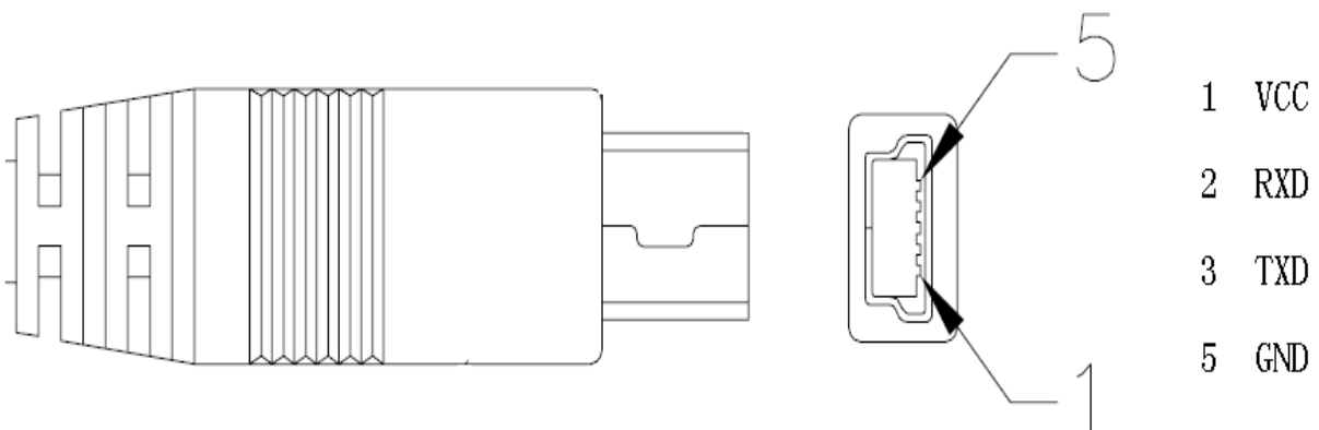
MINI USB Connector
